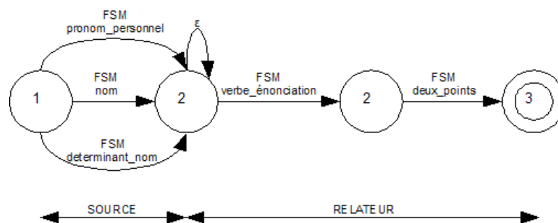
FIG. 1 – Exemple d'un FSM permettant d'associer une expression locuteur avec un relateur.
